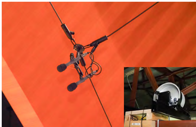
電動吊マイク装置
