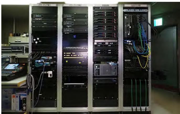
音響調整室 パワーアンプ架、入出力パッチ架
