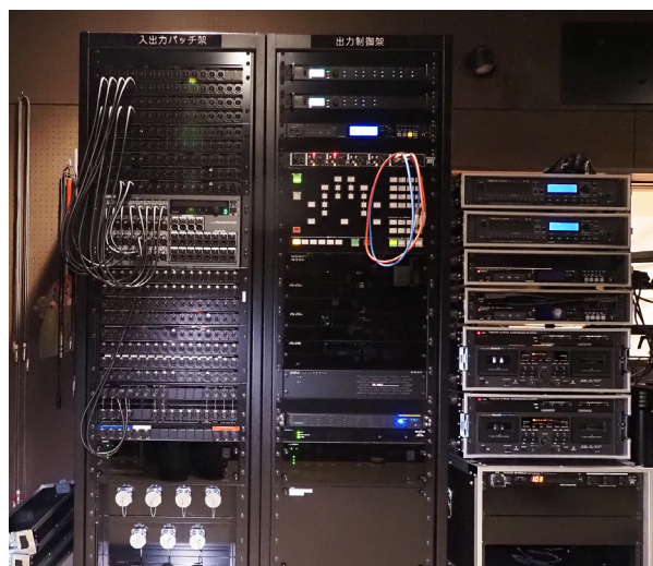
音響調整室 入出力パッチ架 出力制御架
